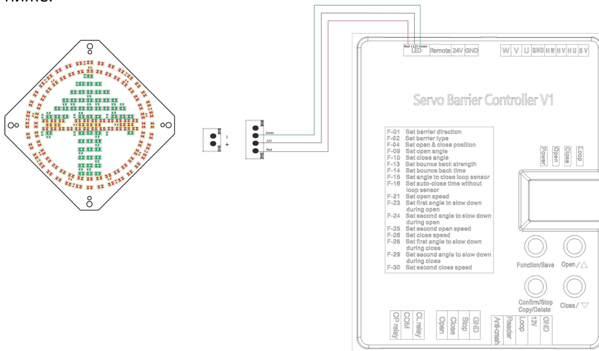
Рисунок 2-46 Подключение к индикатору открытия (стрелка)
