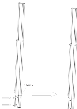
Рисунок 2-22 Установка крепления
