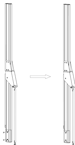
Рисунок 2-34 Установка крепления
