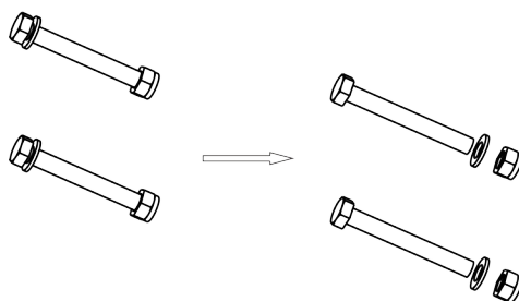
Рисунок 2-5 Монтажные болты
