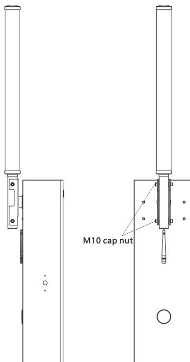
Рисунок 2-16 Установка стрелы
