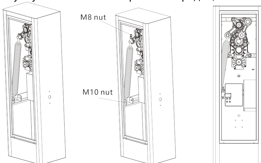
Рисунок 4-1 Замена пружины
