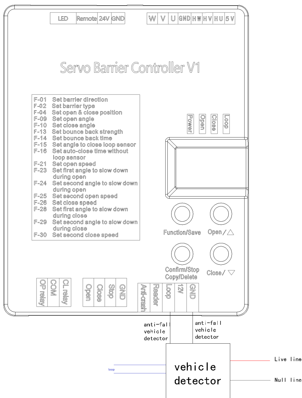
Рисунок 2-43 Подключение к датчику обнаружения ТС
