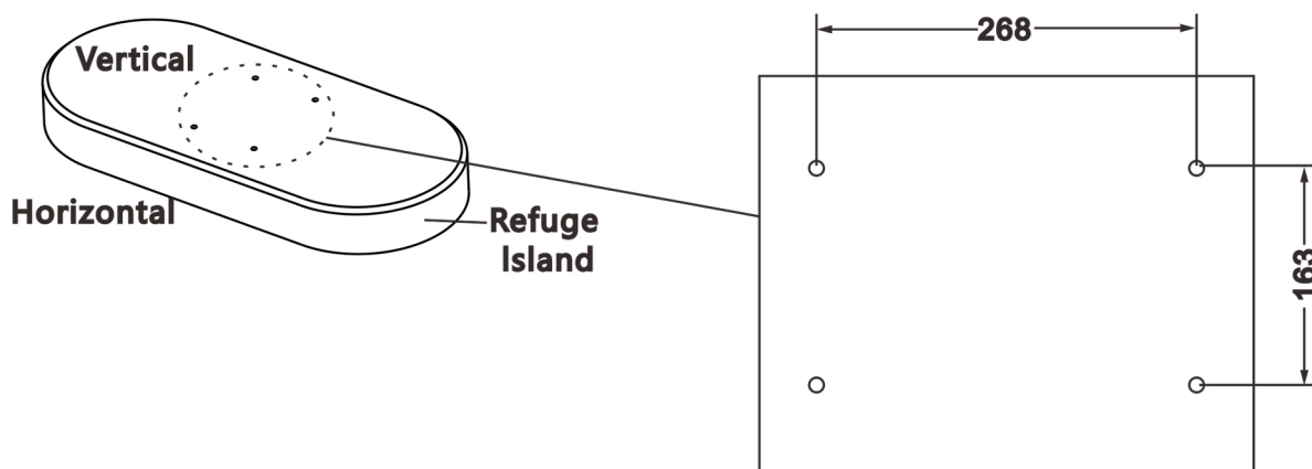
Рисунок 2-1 Расположение отверстий
