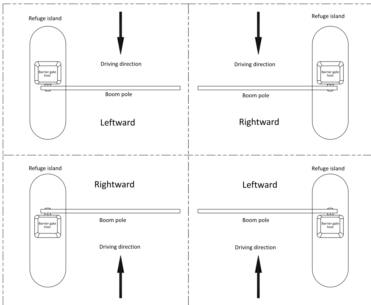
Рисунок 4-3 Инструкция по выбору направления стрелы
