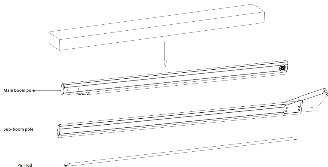
Рисунок 1-9 Складная стрела
