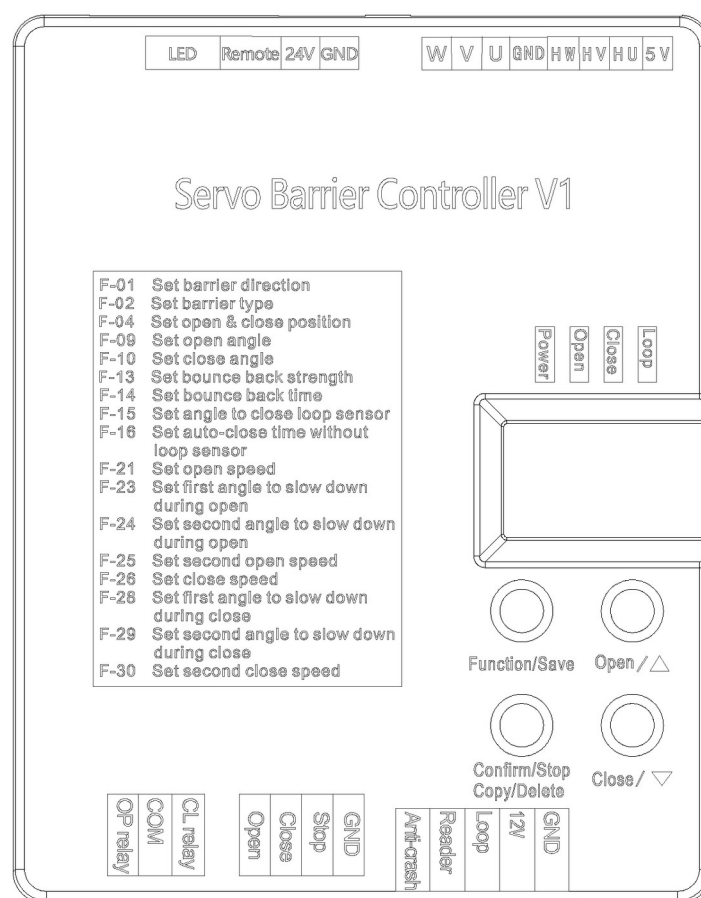
Рисунок 3-1 Кнопки управления
