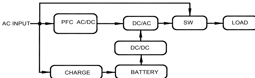
Рис.3.1-1 Блок-схема ИБП серии Monolith K 1к - 3к
