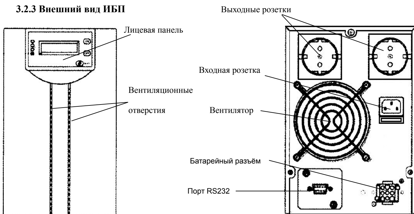
Рис.3.3-2 Внешний вид ИБП Monolith K 1к
