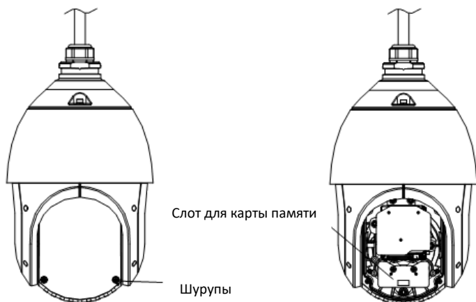
Рисунок 2-2 Установка SD-карты
