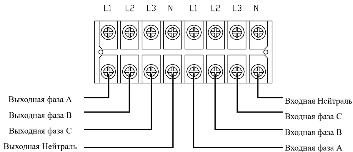
Рис. 2-3-1 Блок клемм ИБП ХЕ 10 / 20
