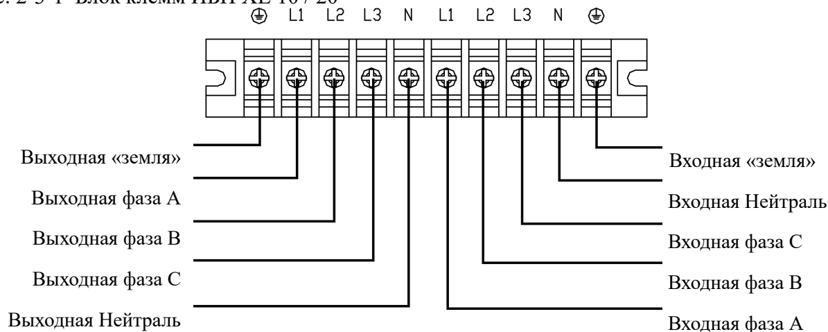
Рис.2-3-2 Блок клемм ИБП ХЕ 10WB / 20WB
