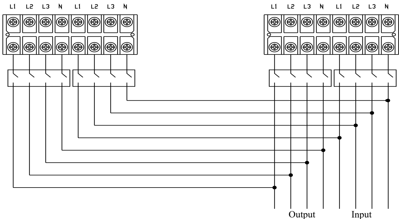
Рис.2-4-1 Подключение в параллельную систему ИБП ХЕ 10 / 20 ( на примере двух ИБП).
