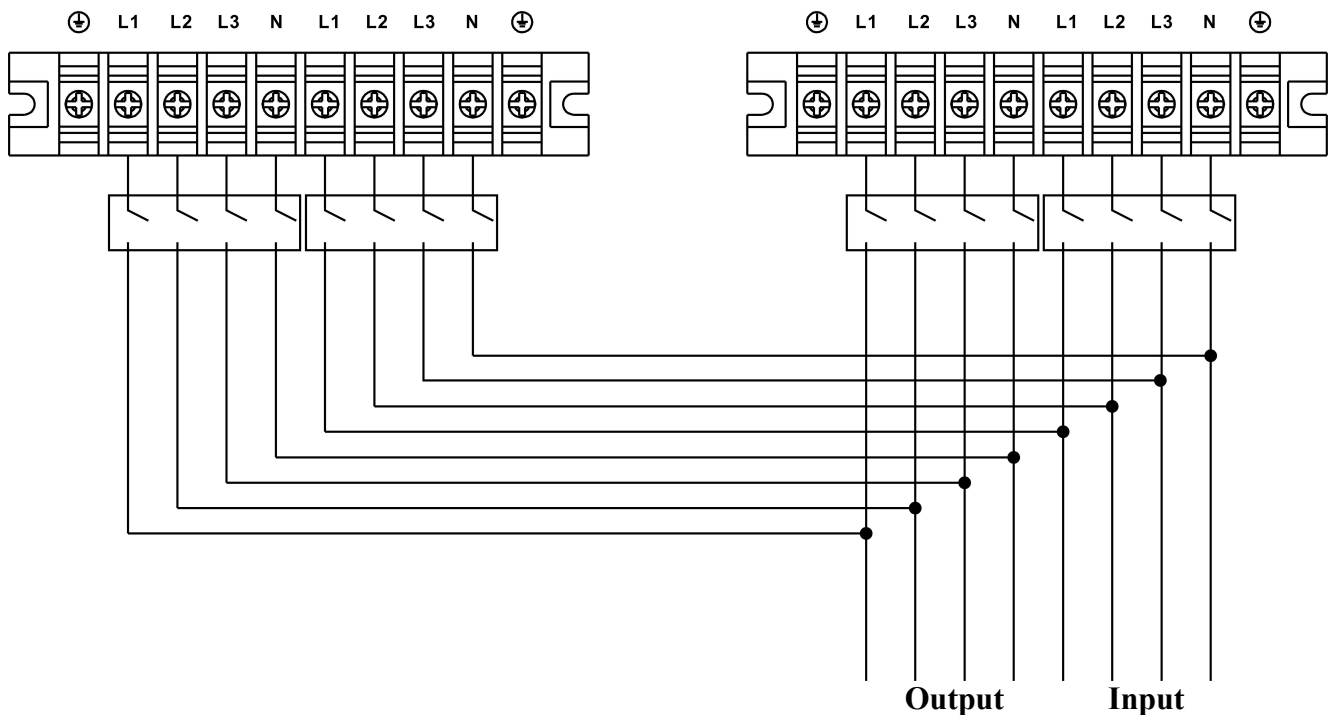
Рис.2-4-2 Подключение в параллельную систему ИБП ХЕ 10WB/ 20WB (на примере двух ИБП).
