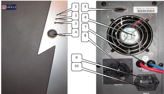
Лицевая панель ИБП
