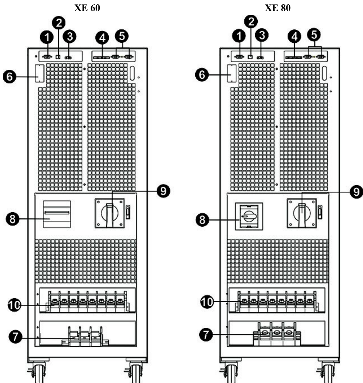
Рис.2-2-2 Внешний вид задней панели ИБП.
