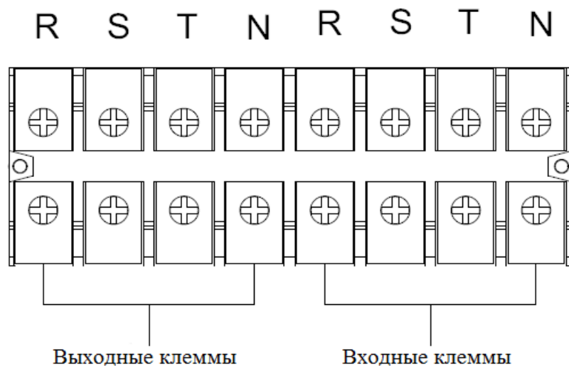
Рис. 2-3-1 Блок клемм ИБП ХЕ 30(WB) / 40(WB)
