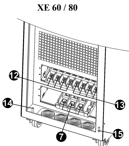
Рис.2-2-1 Блок клемм для подключения ИБП
