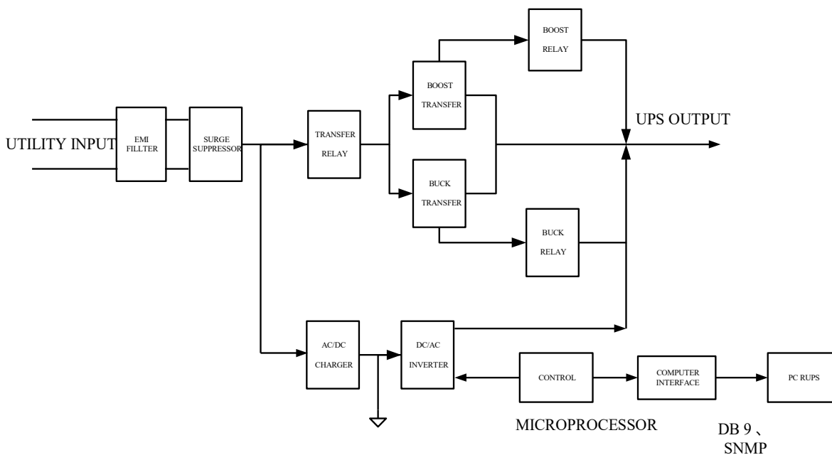
Рис.3.1-1 Блок-схема ИБП
