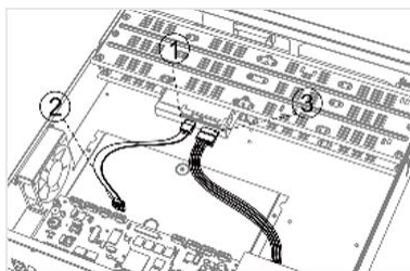
Рисунок 1-3 Подключение кабелей
