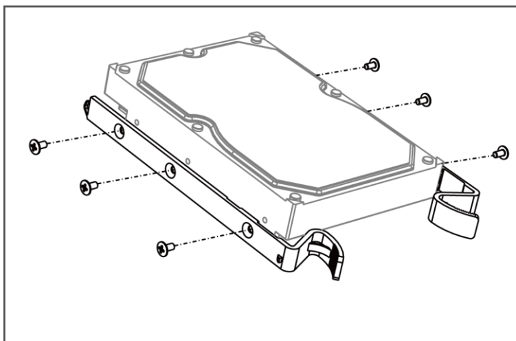
Рисунок 1-4 Фиксация монтажных проушин на HDD
