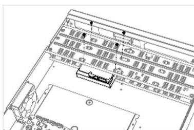
Рисунок 1-2 Фиксация HDD
