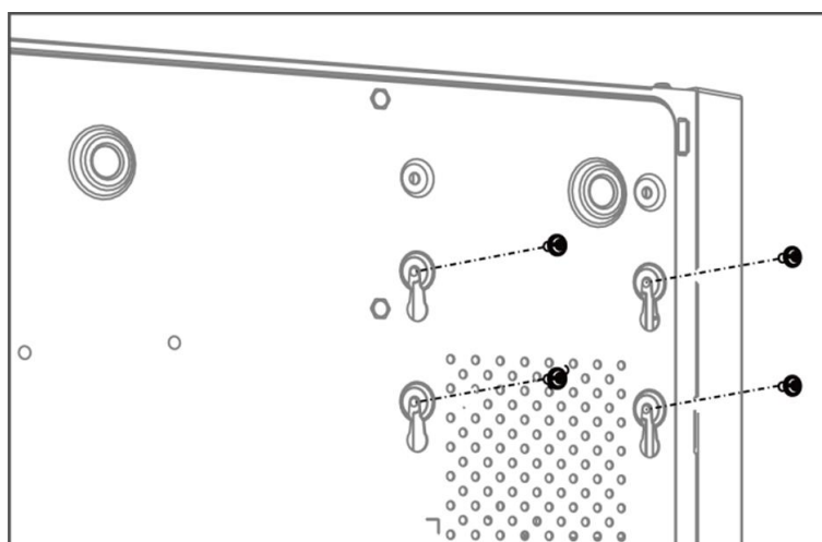
Рисунок 1-11 Фиксация HDD на нижней панели устройства
