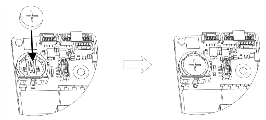
Рисунок 1-2 Замена батареи
