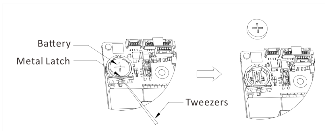
Рисунок 1-1 Извлечение батареи
