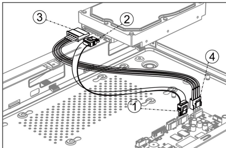
Рисунок 1-10 Подключение кабелей
