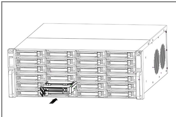
Рисунок 1-8 Установка корпуса HDD в слот
