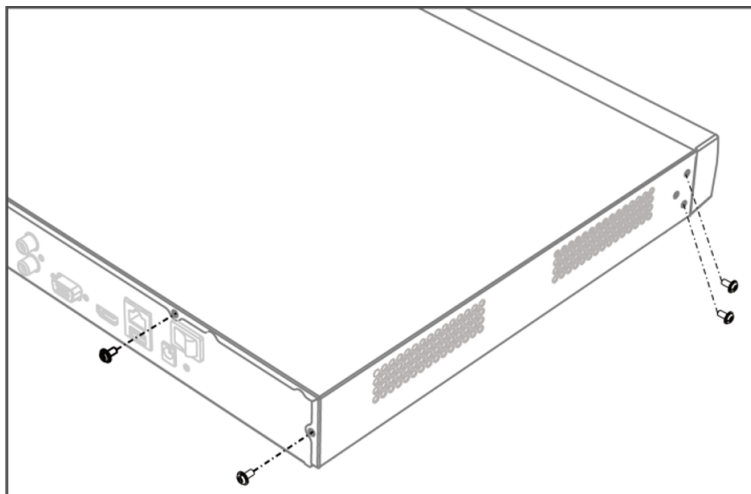
Рисунок 1-9 Снимите крышку
