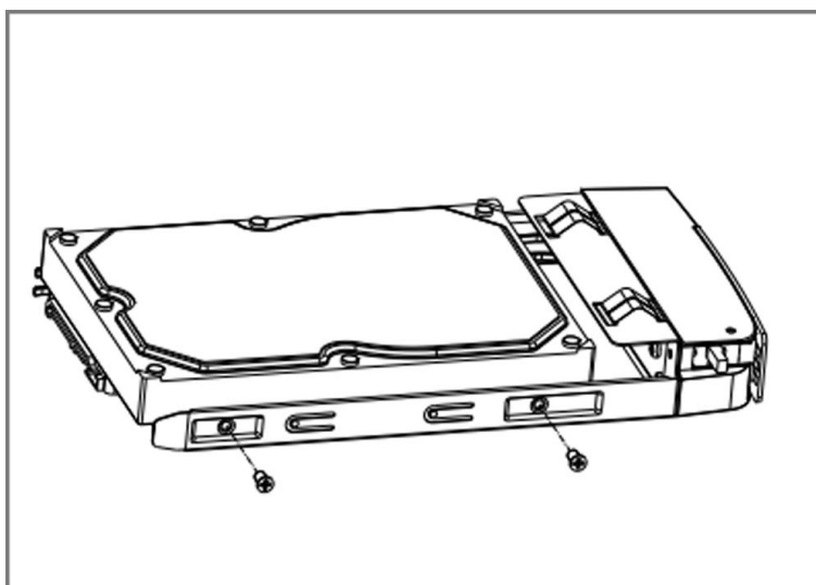
Рисунок 1-7 Фиксация HDD
